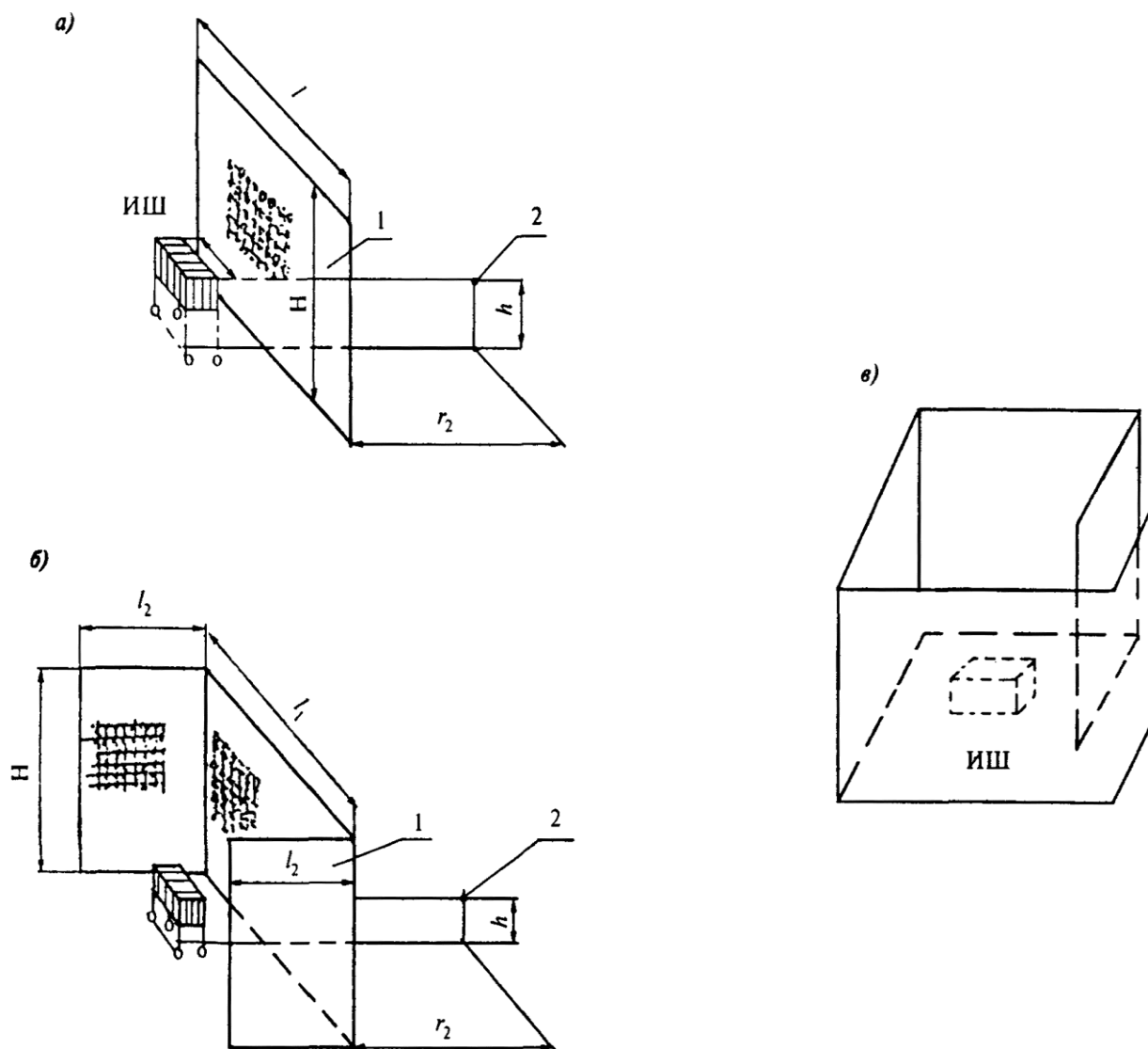
а - плоский; б - П-образный; в - выгородка; ИШ - источник шума; 1 - экран; 2 - расчетная точка
