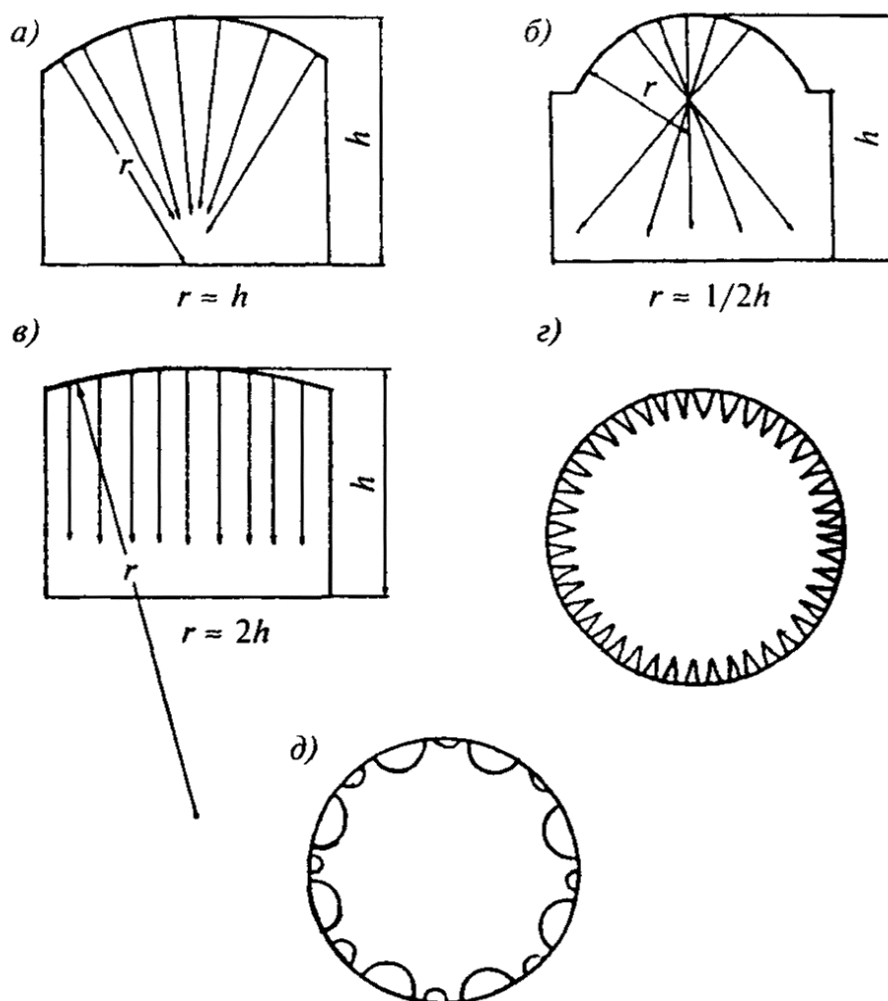
Рисунок 9 - Варианты решения зала с куполом
