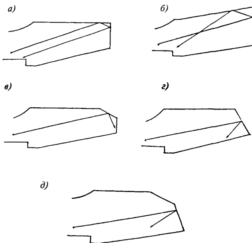
Рисунок 7 - Оформление портала, позволяющее направить первые отражения в глубину зала
