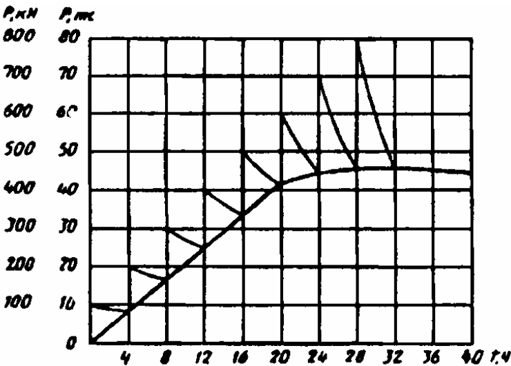
Рисунок 1 - График изменения нагрузки P во времени T
