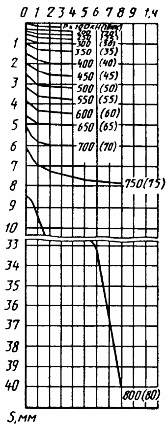
График изменения осадки сваи S во времени (по ступеням нагружения)
