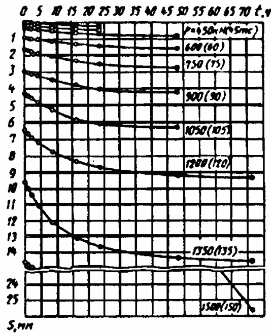
График изменения осадки сваи S во времени T (по ступеням нагружения)
