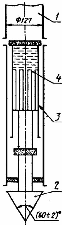
Схема конструкции сваи- зонда
