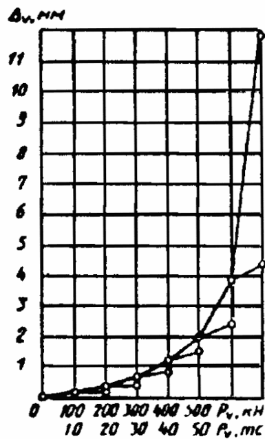
График изменения выхода сваи из грунта \Delta v во времени T (по ступеням нагружения)
