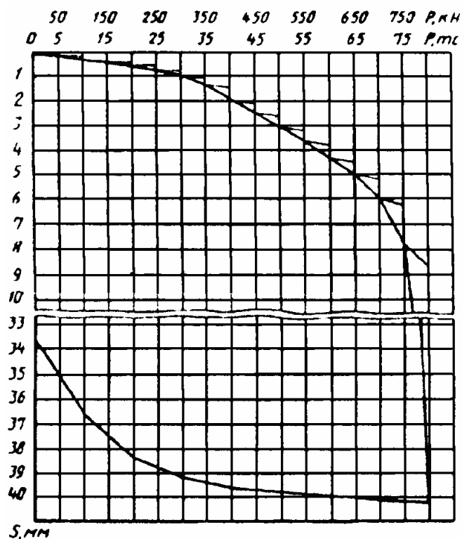
График изменения осадки сваи S во времени (по ступеням нагружения)
