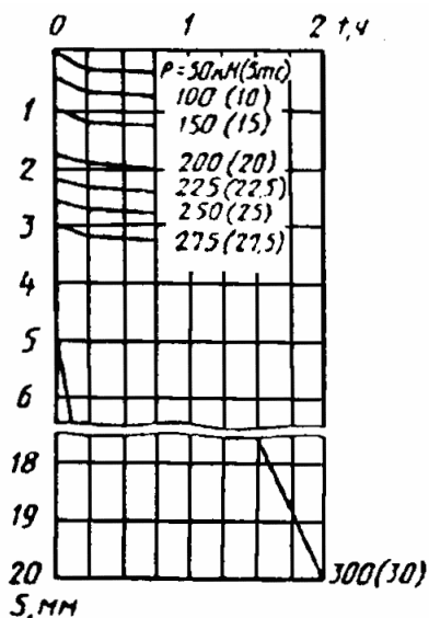
График изменения осадки свай S во времени T по ступеням нагружения)
