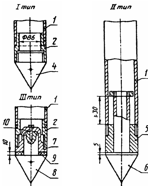
Схемы конструкций эталонной сваи Нижняя часть с наконечником
