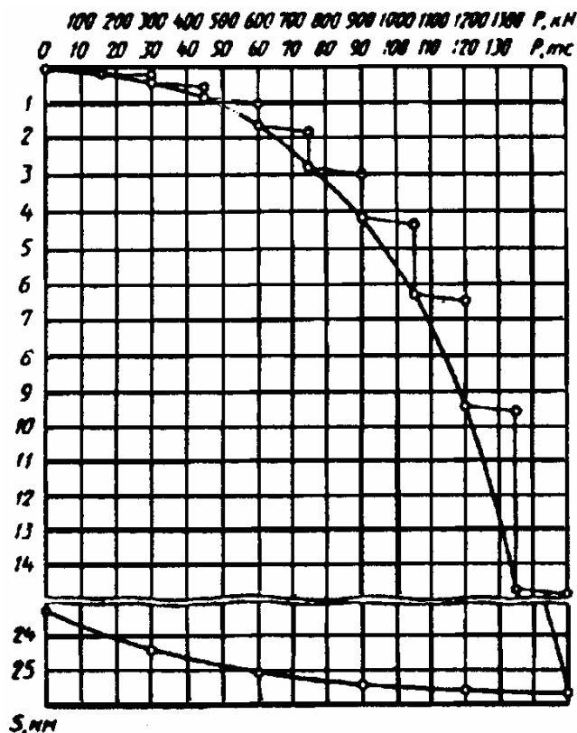
График зависимости осадки сваи S от нагрузки P
